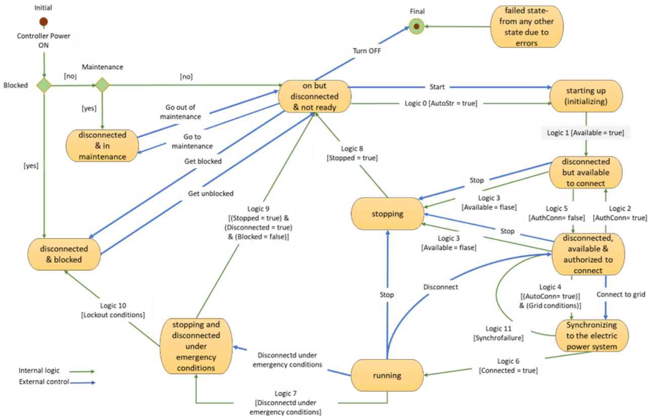
Figure 2 : Diagramme générique de l'état opérationnel réel et de connexion d'un DER comme décrit dans IEC 61850-7-420
