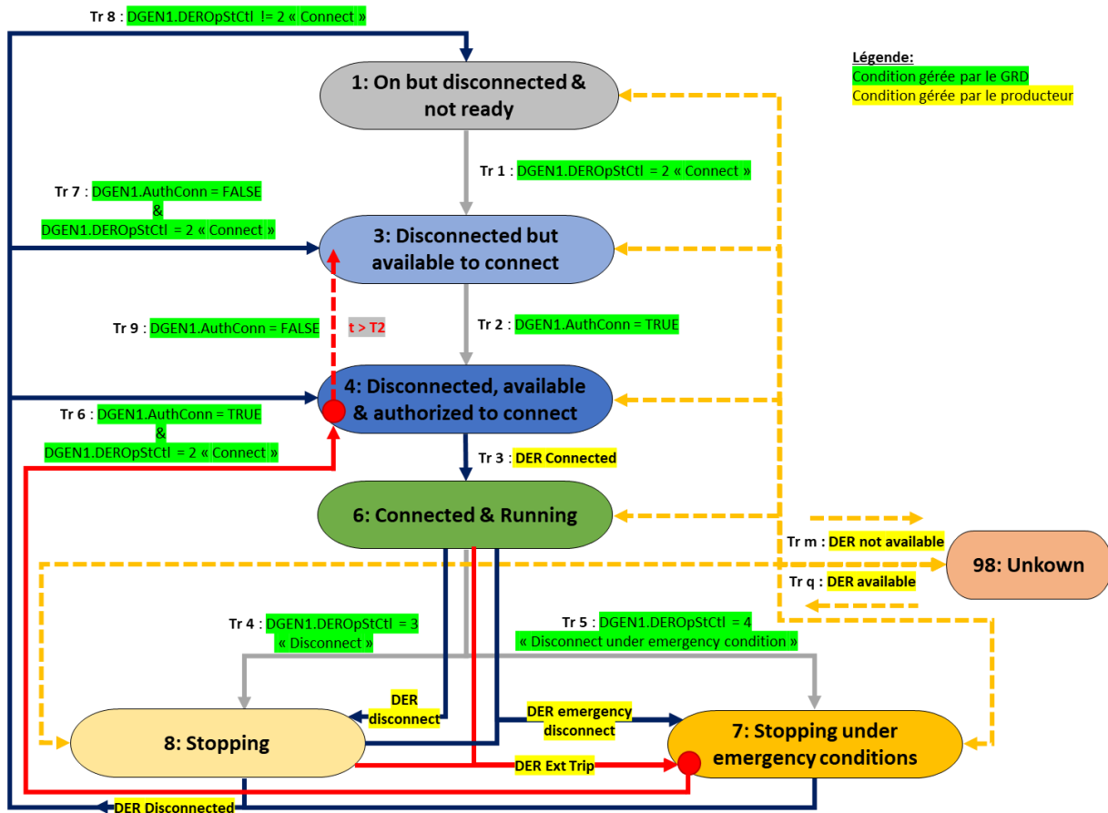
Figure 3 : Diagramme de de gestion de connexion d'un producteur HTA du point de vue conduite d'EDF SEI
