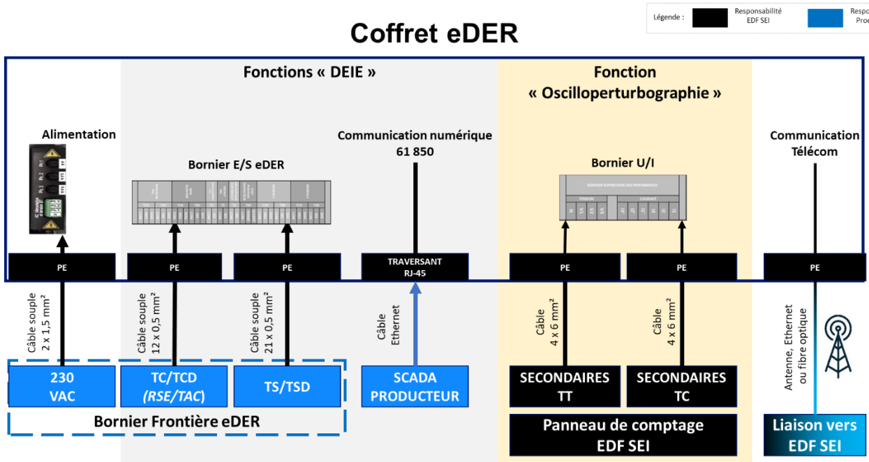
Schéma de principe de l'eDER
